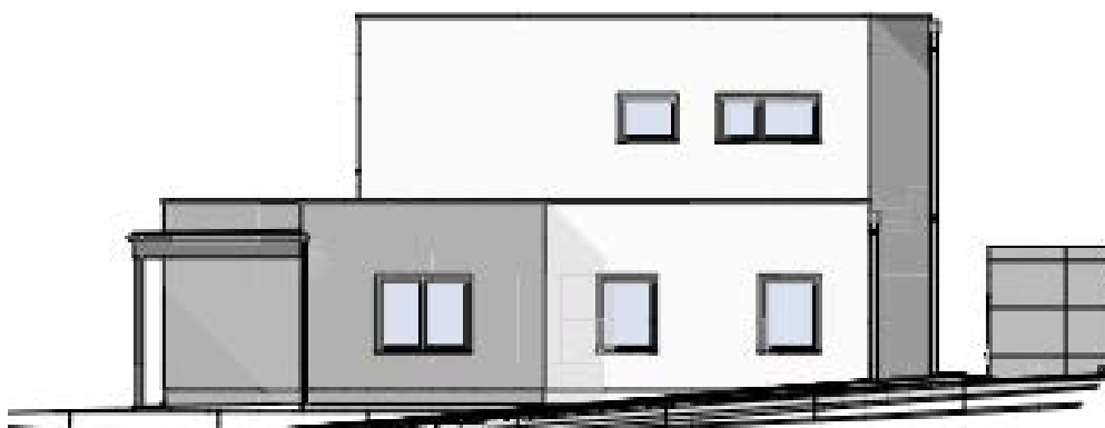
OST – ANSICHT
